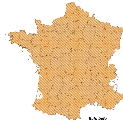
Bufo bufo
